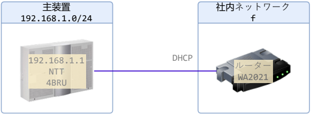
論理構成図
